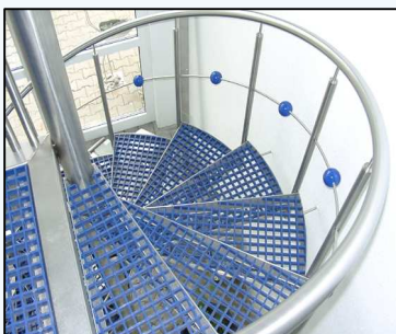
GFK Gitterroste
